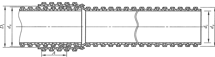
图 2 典型的弹性密封圈连接示意图
