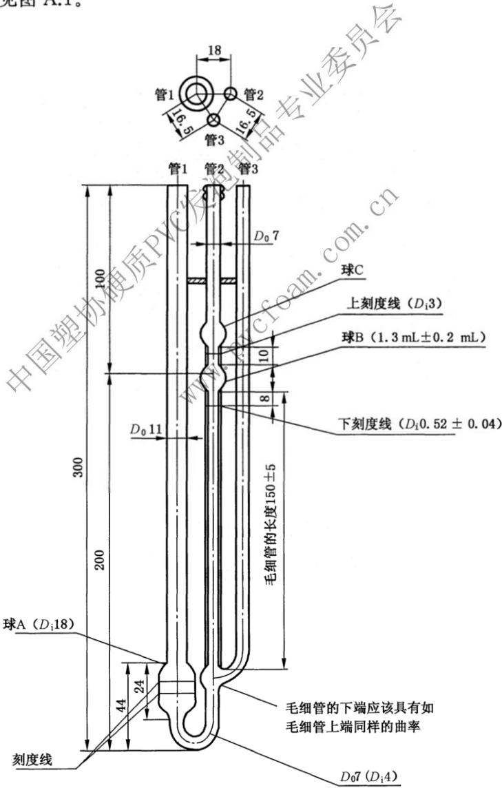
图 A.1 乌式黏度计示意图
