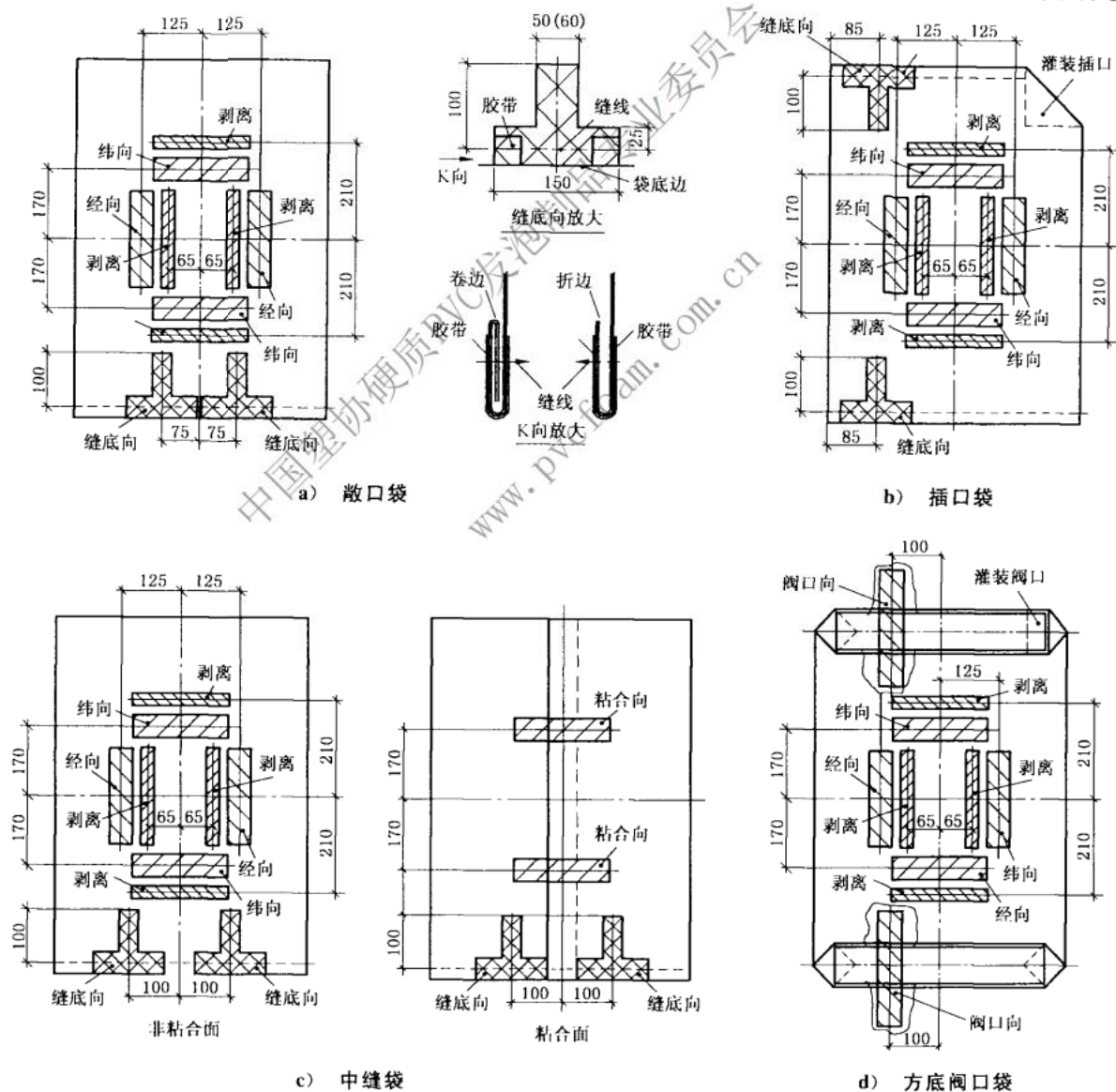
图 C.1 取样位置图
